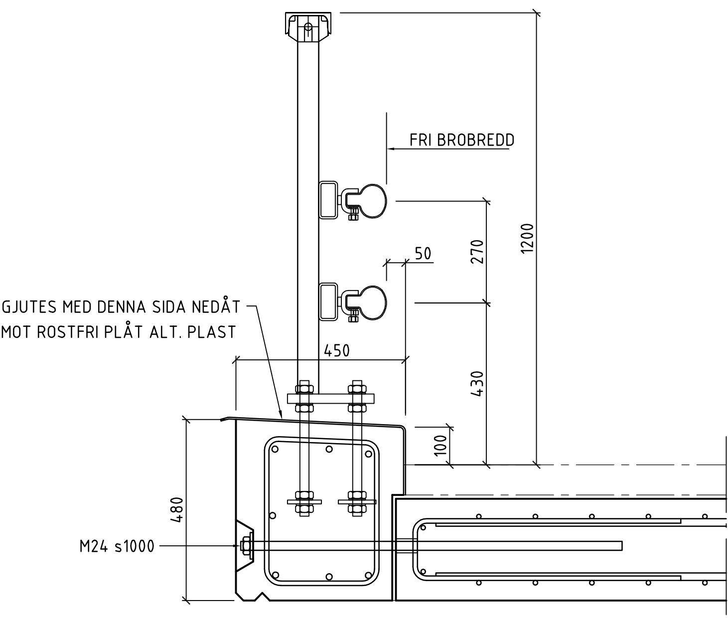
SEKTION
