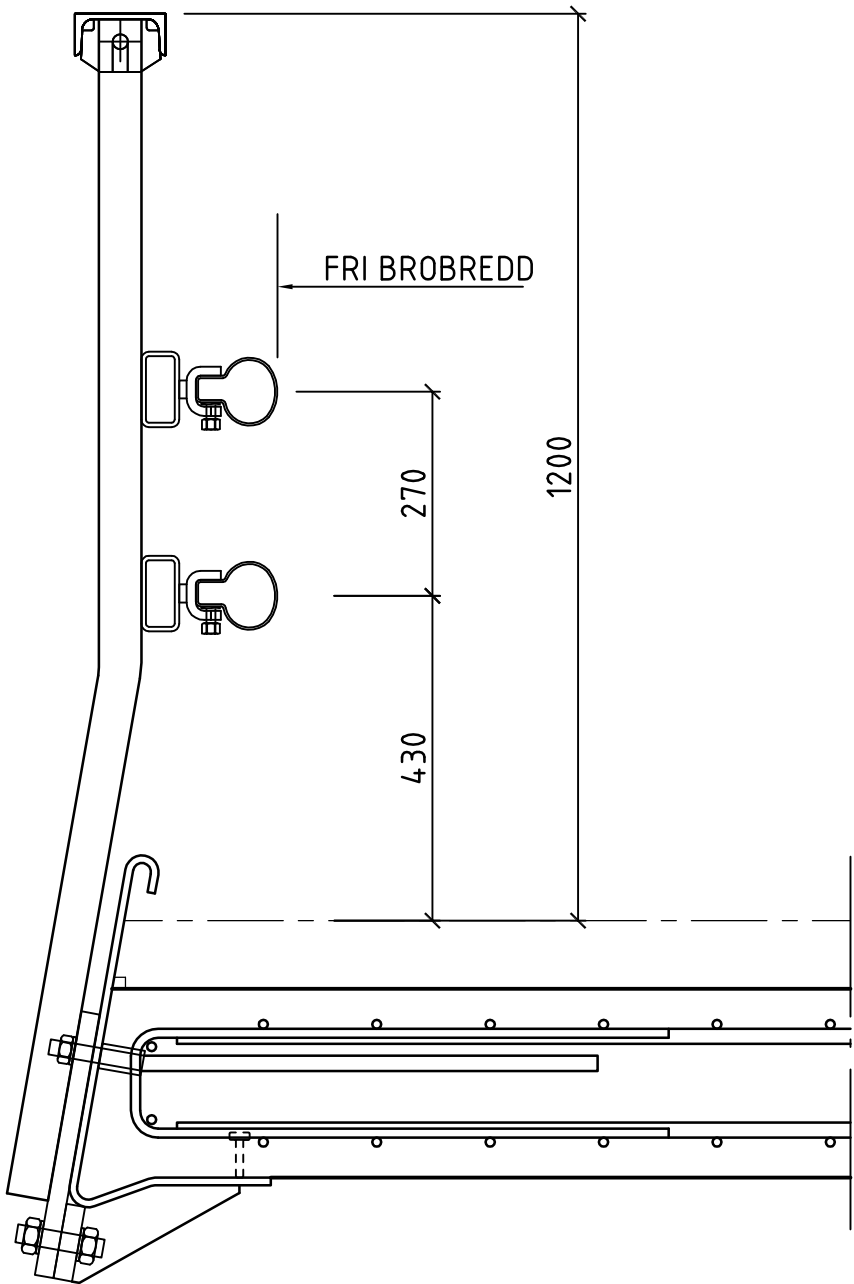
SEKTION
