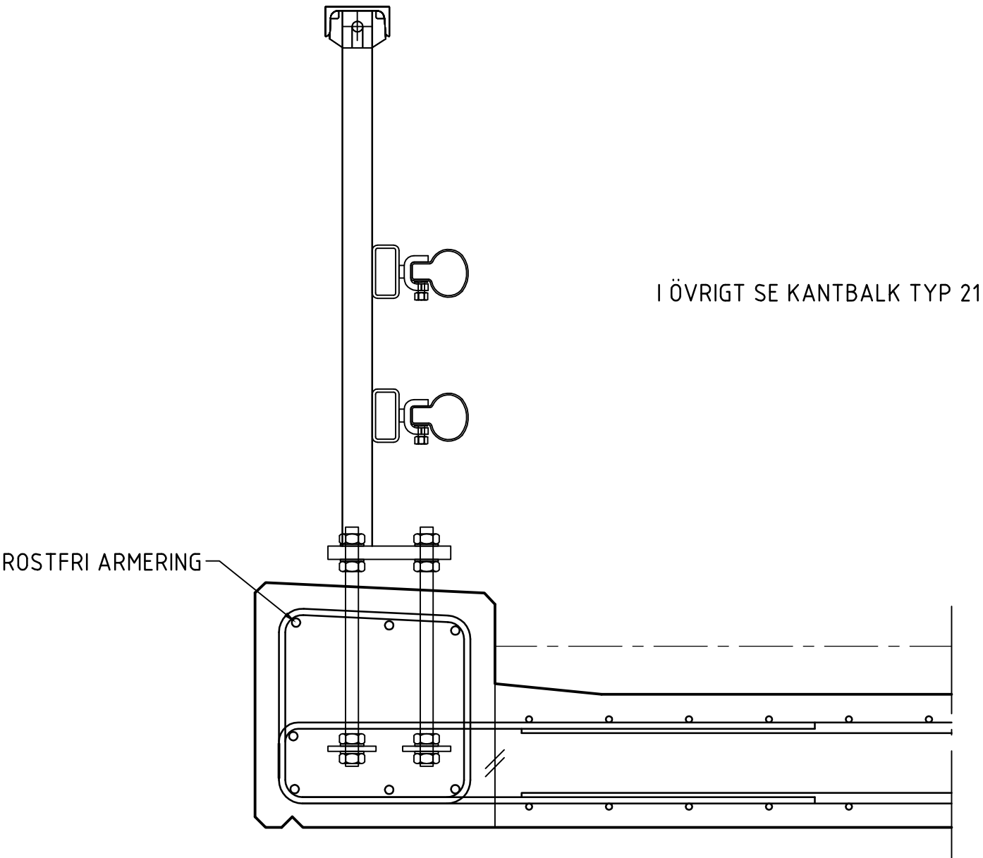
SEKTION
