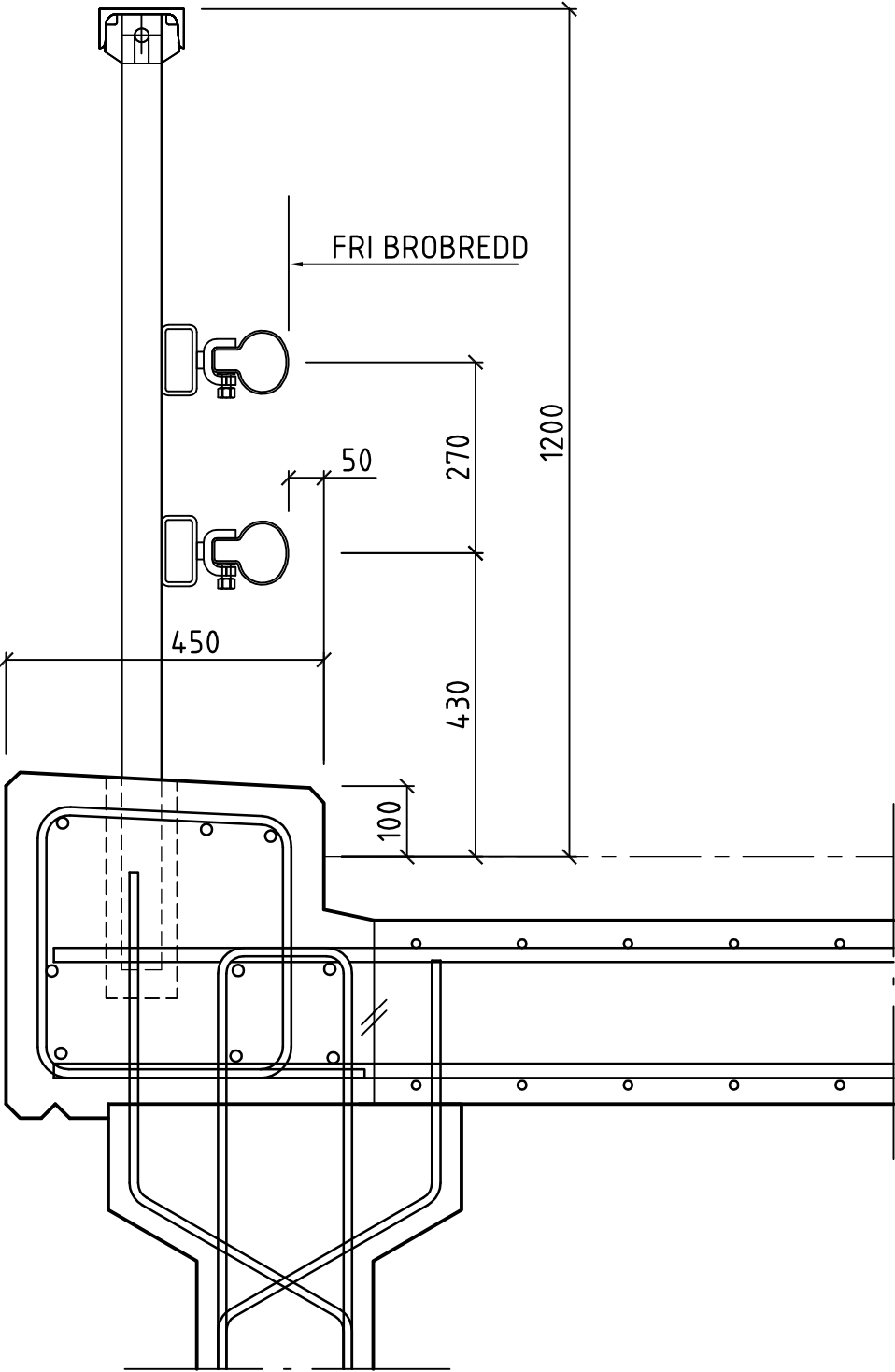
SEKTION
