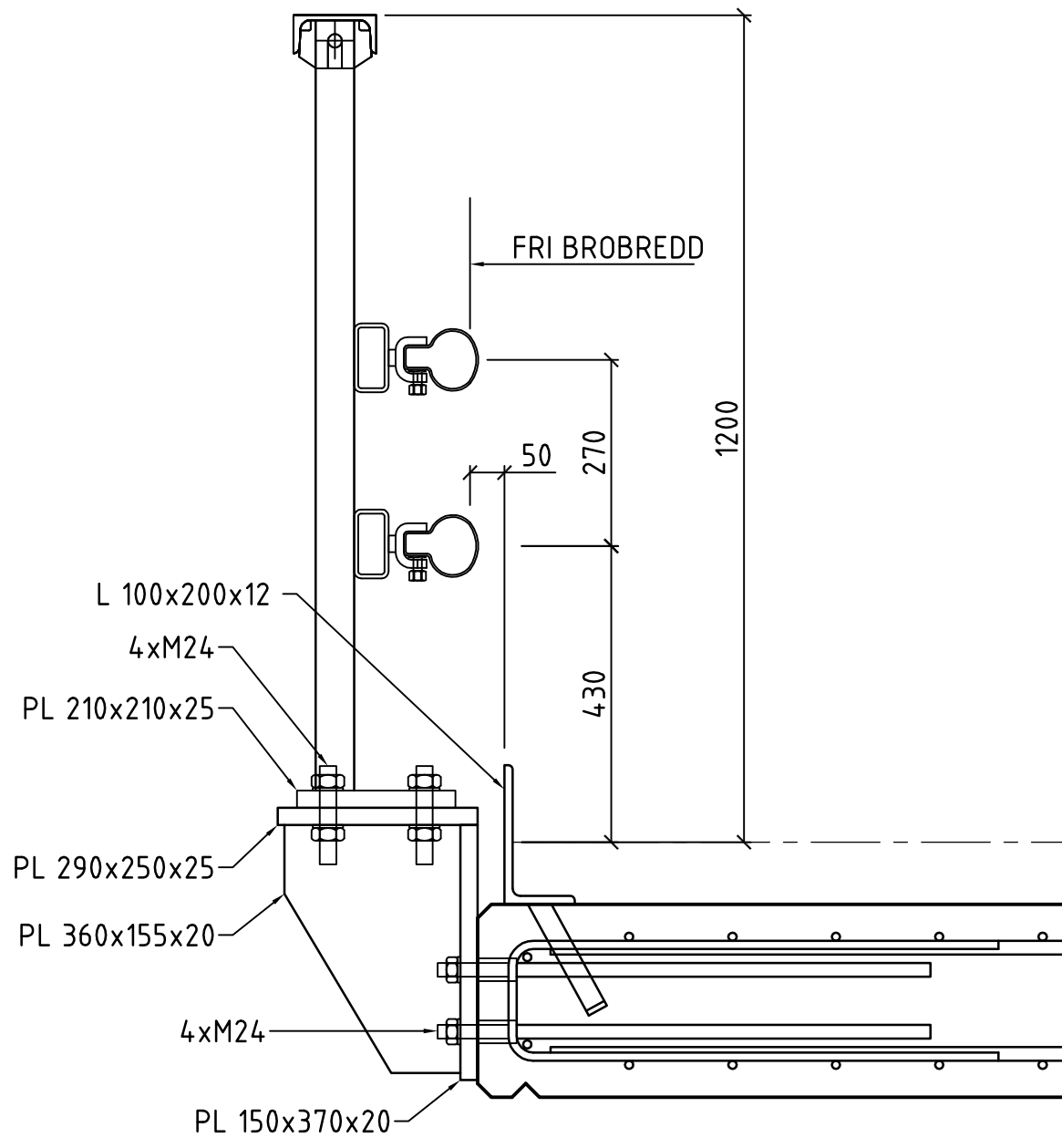
SEKTION
