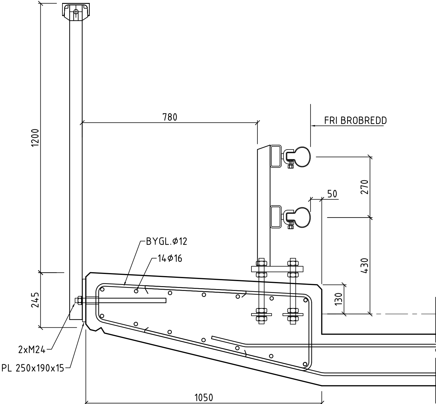
SEKTION
