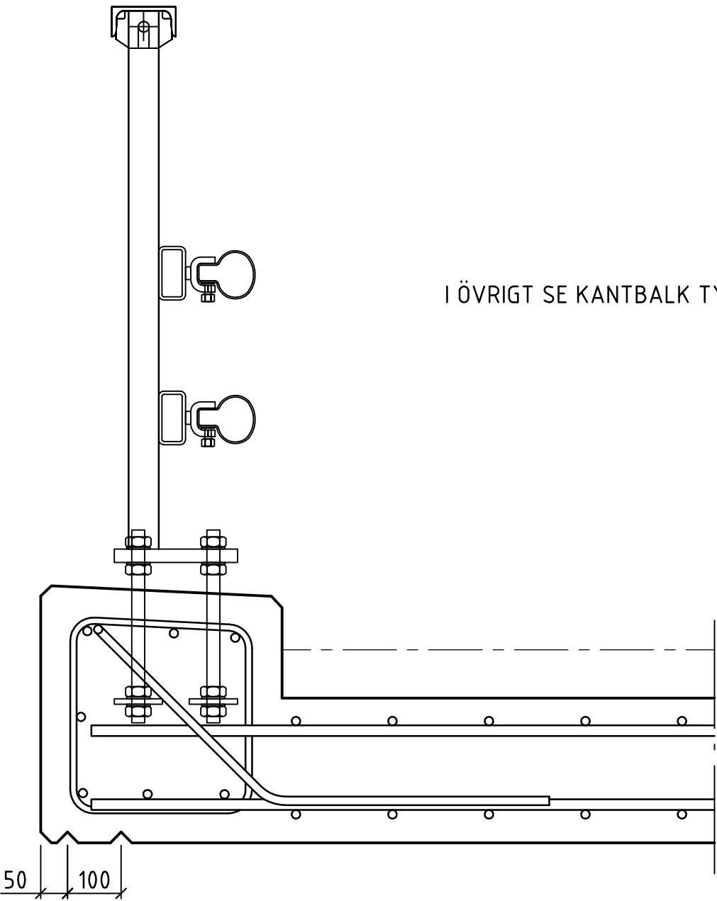
SEKTION
