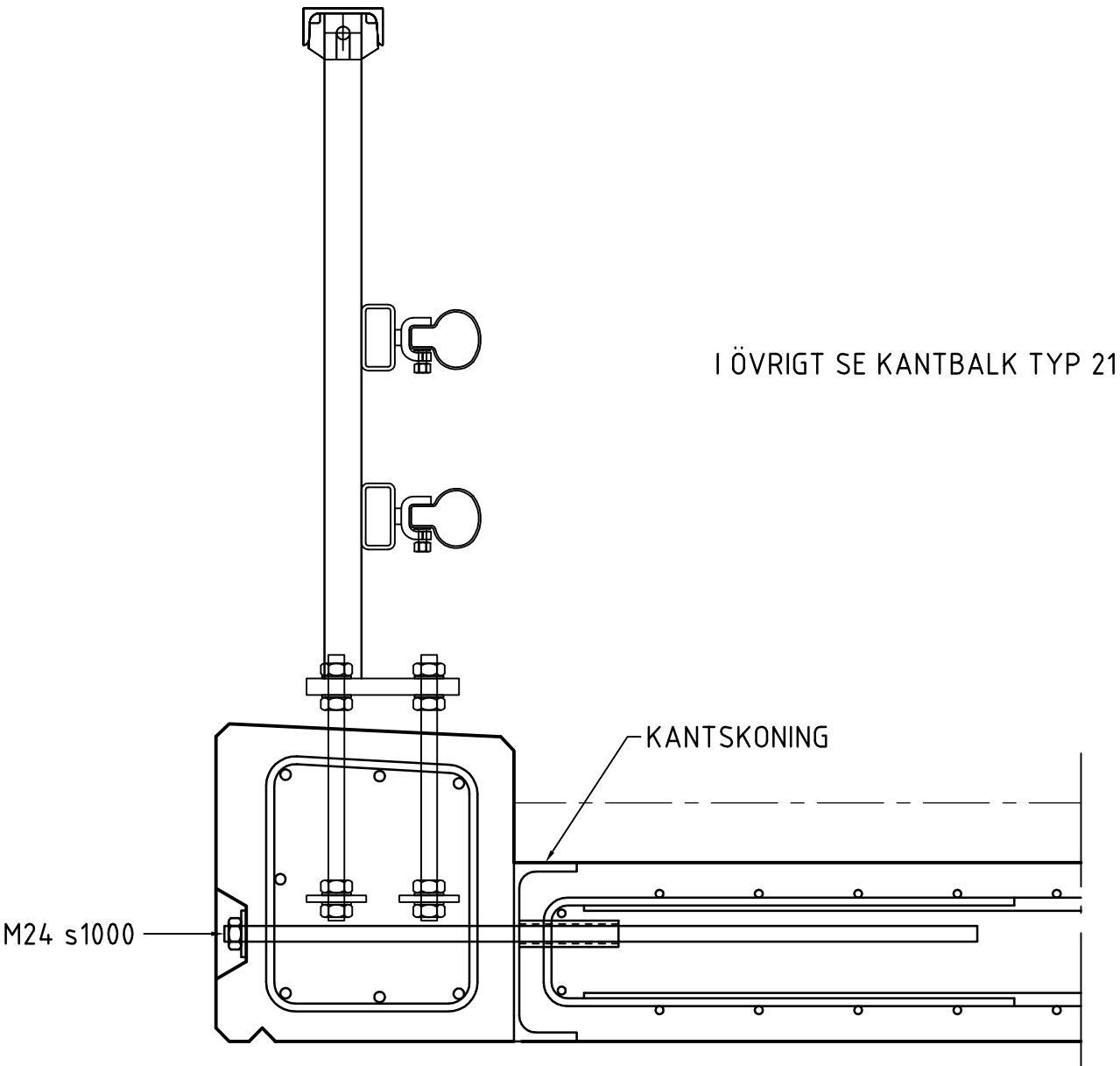
SEKTION
