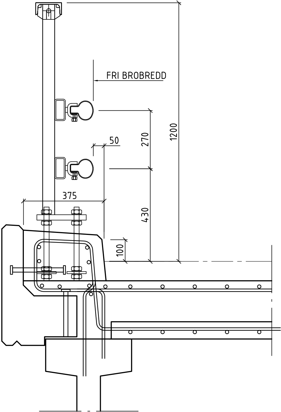
SEKTION
