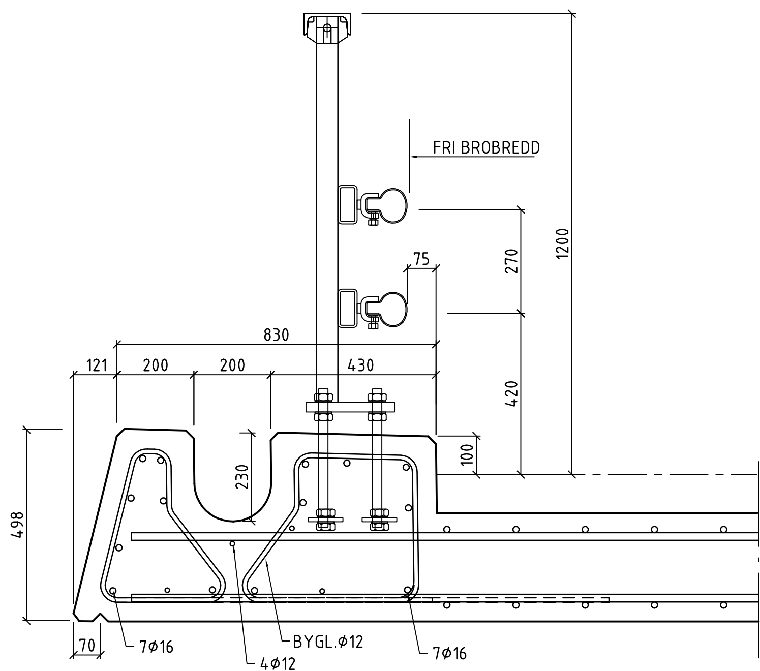
SEKSION
