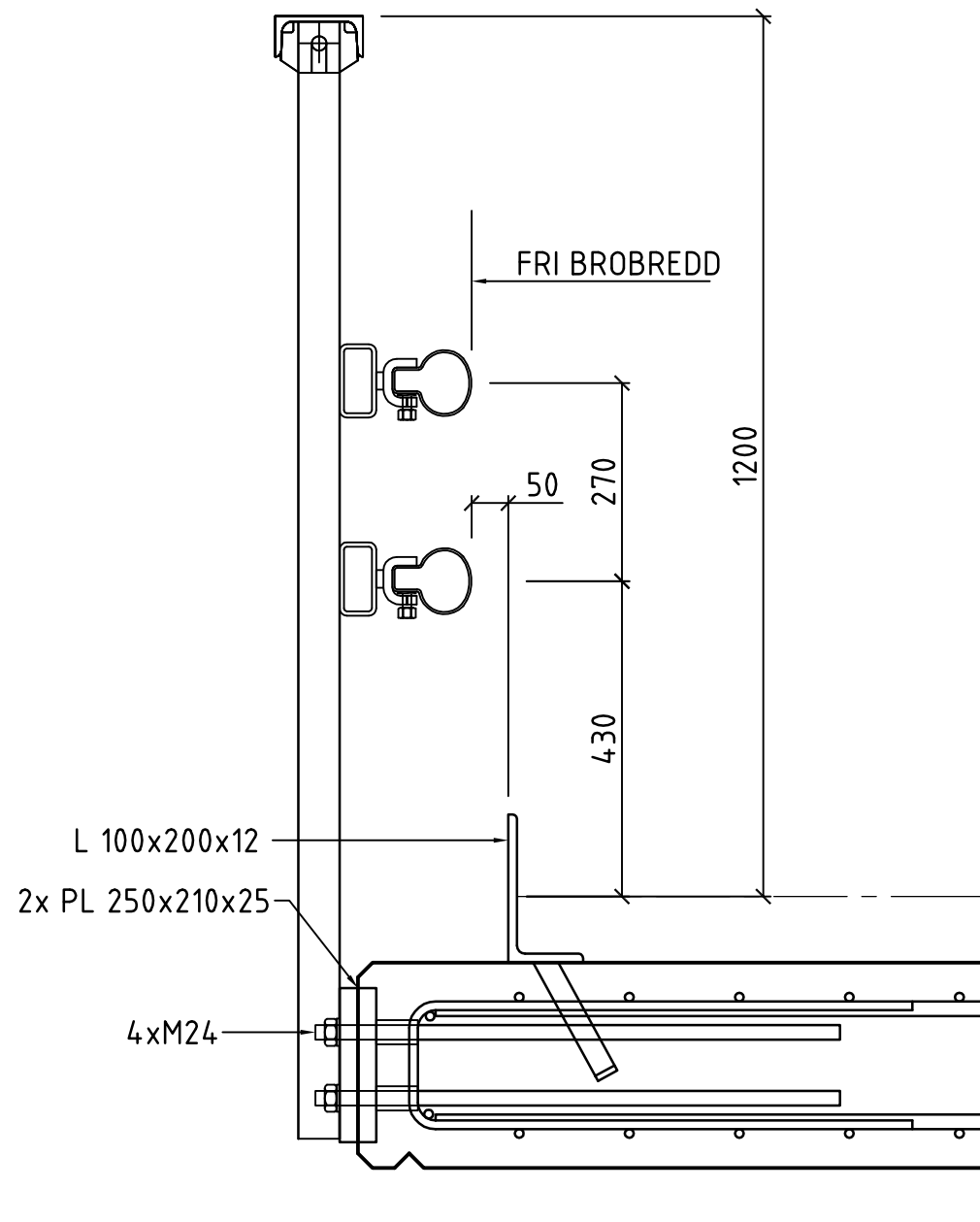
SEKTION
