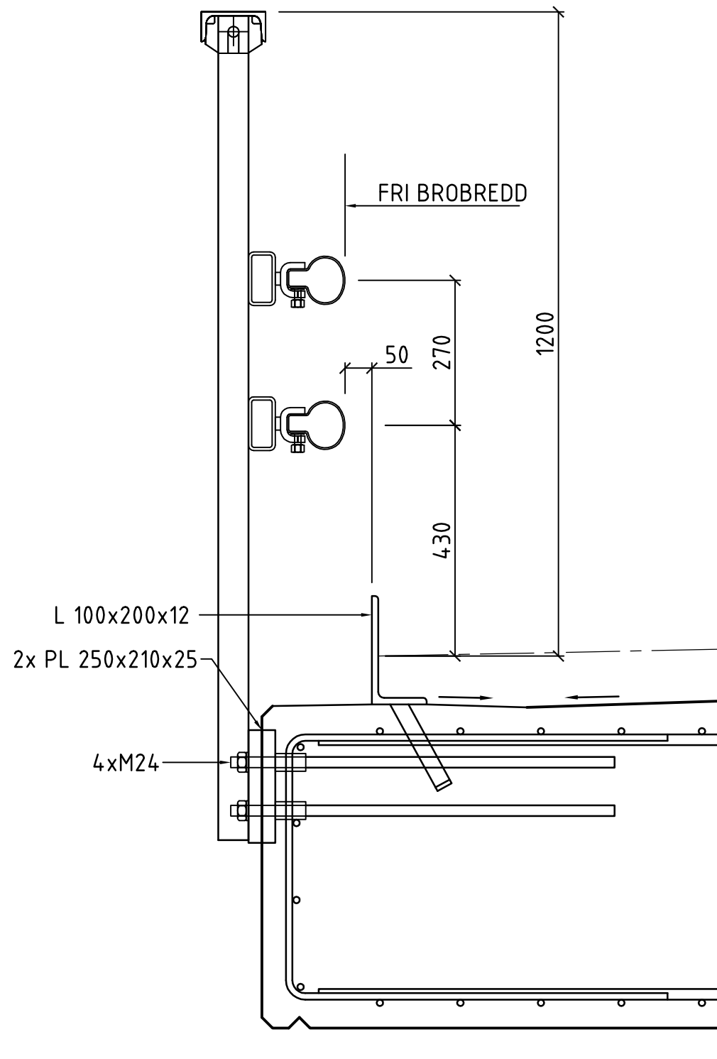
SEKTION
