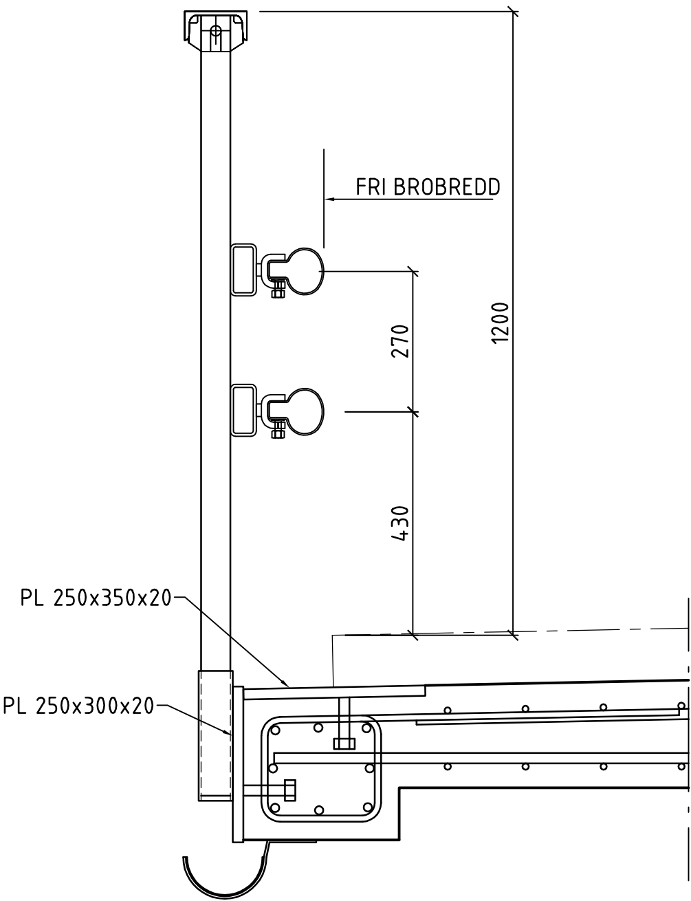
SEKSION
