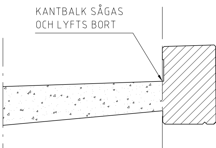
STEG 1 1:20
