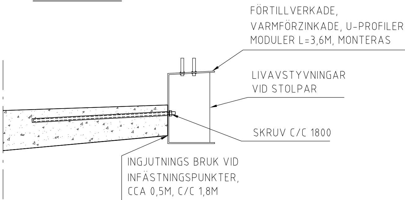
STEG 3 1:20
