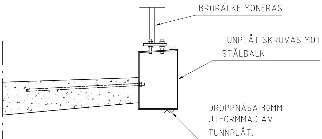
STEG 4 1:20
