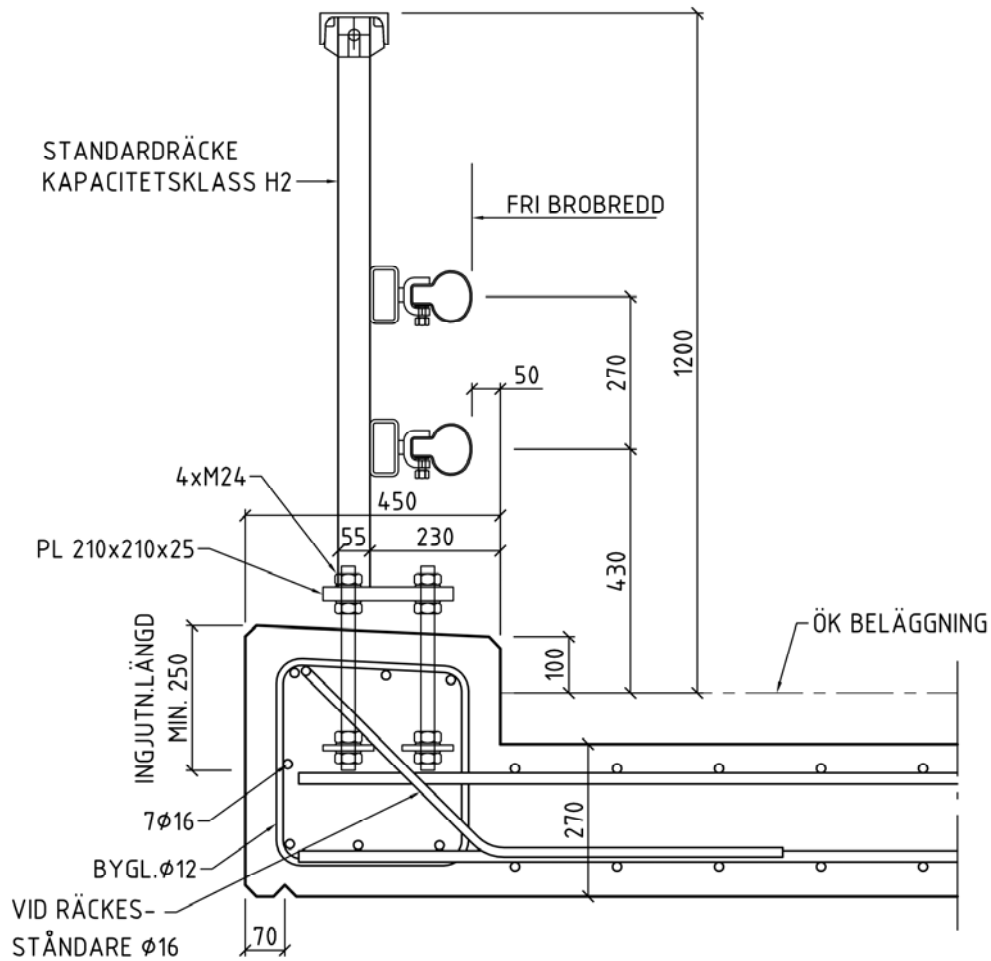
Figur 21.1 a) Kantbalk typ 21, sektion
