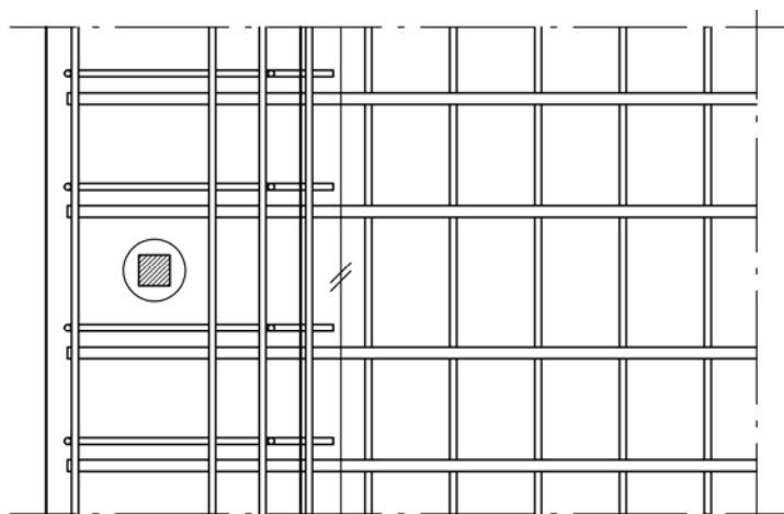
Figur 16.1 a) Kantbalk typ 16, sektion
