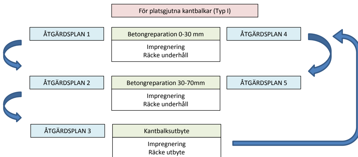
Figur 6.13 Exempel av en åtgärdsplan för platsgjutna kantbalkar. I grön visas "Master"-aktivitet och med de följande "Slav" i vitt.
