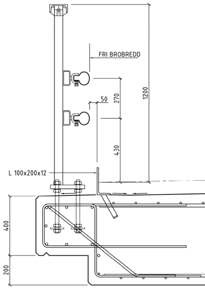
Figur 7.1 a) Kantbalk typ 7, sektion.
