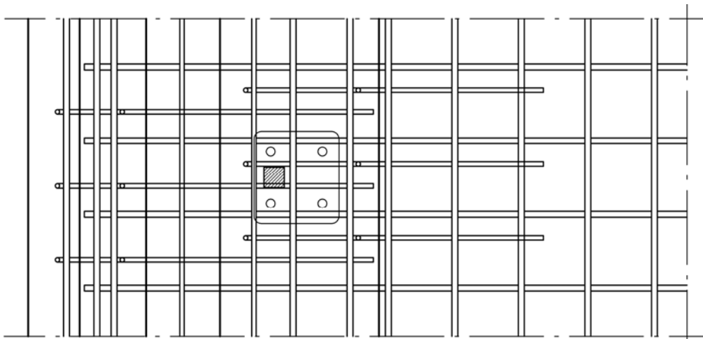
Figur 23.1 a) Kantbalk typ 23, sektion
