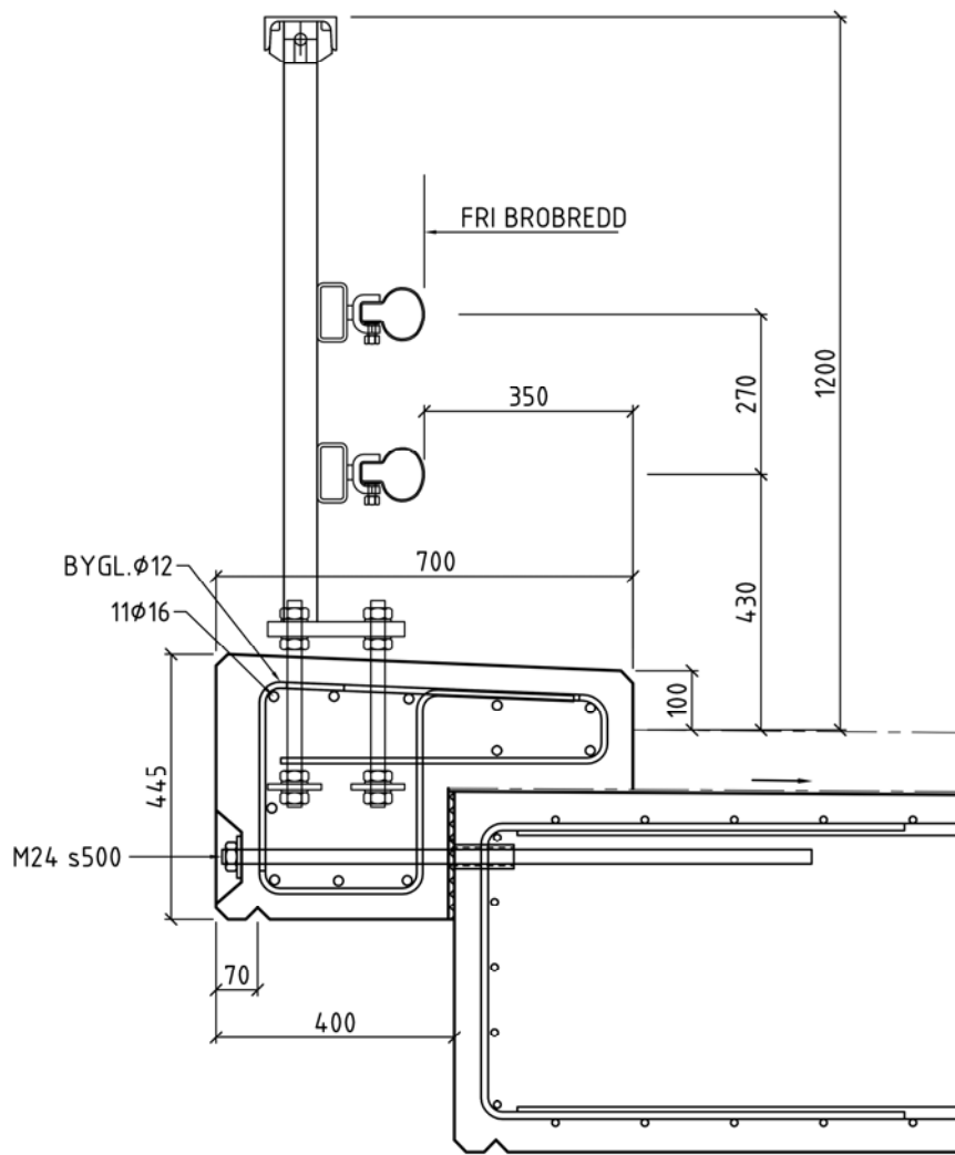
Figur 14.1 a) Kantbalk typ 14, sektion
