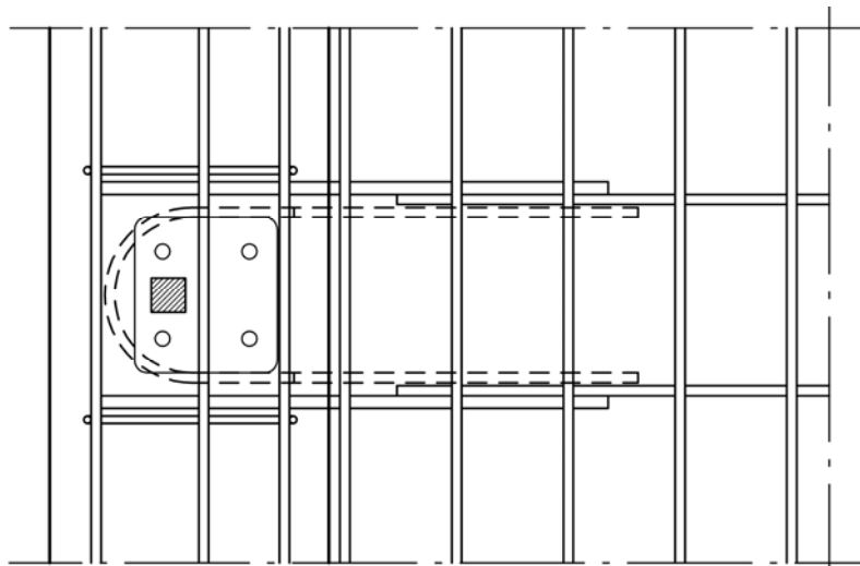
Figur 21.1 b) Kantbalk typ 21, plan.
