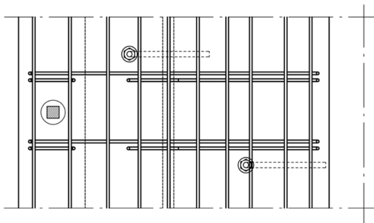
Figur 12.1 b) Kantbalk typ 17, plan.
