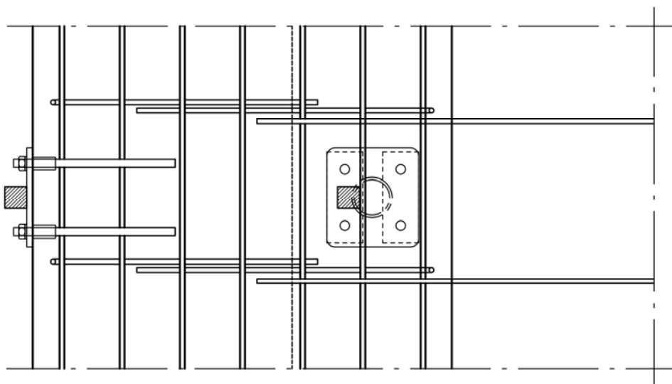
Figur 20.1 a) Kantbalk typ 20, sektion
