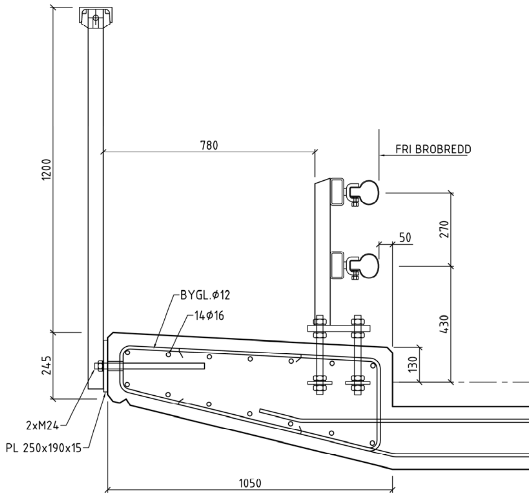
Figur 20.1 a) Kantbalk typ 20, sektion
