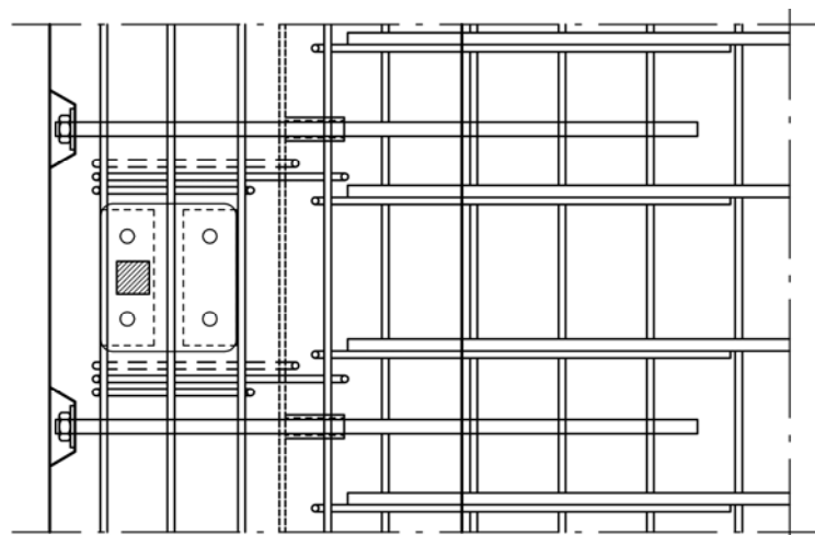
Figur 14.1 a) Kantbalk typ 14, sektion
